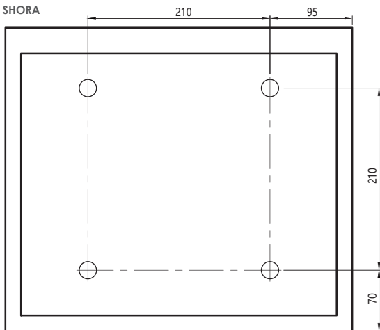
POHLED ZEPŘEDU
