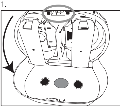
Ouvrir le distributeur à l'aide du bouton-poussoir de verrouillage situé sur le dessous du distributeur
