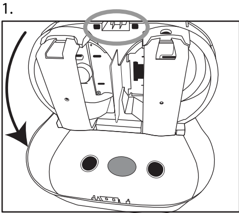
เปิดเครื่องจ่ายโดยใช้ปุ่มกลิ้งล็อคที่อยู่ด้านล่างของเครื่องจ่าย
