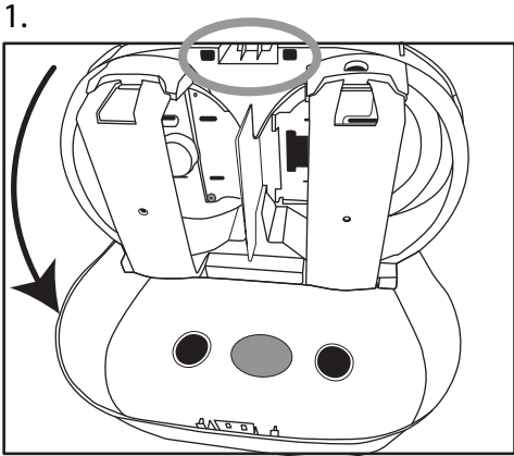
1. 使用衛生紙架外側的壓式快鎖按鈕，開啟衛生紙架
