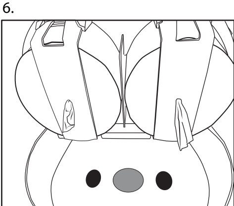
Refermer les supports intérieurs et tirer 2 à 3 feuilles de chaque rouleau pour s'assurer qu'il n'y a aucun bourrage de papier
