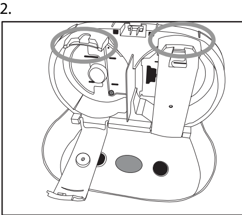
Ouvrir les supports porte-rouleaux internes en soulevant le dessus des supports
